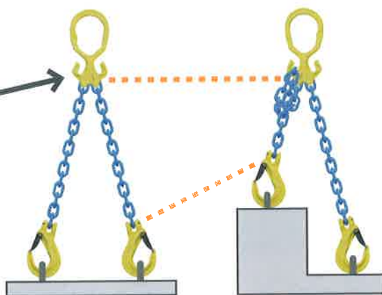
偏荷重物を吊る
